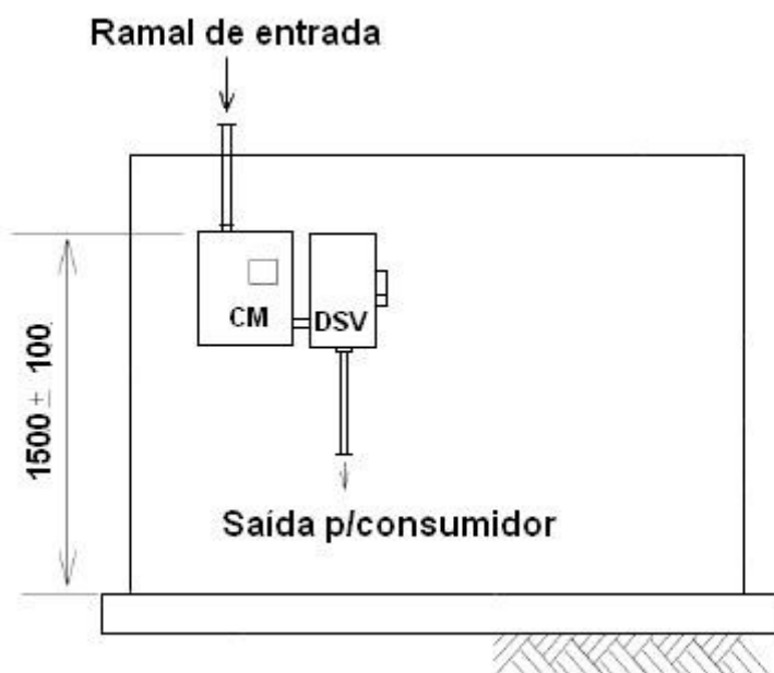
Figura 11 – Instalação de DSV para circuitos sem inversor
